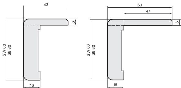
Rohový prvok zárubne SW, S8 obložka standard
