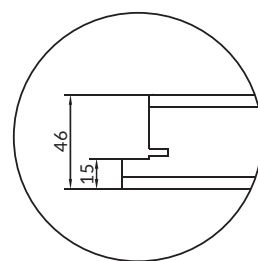
rez dverí
