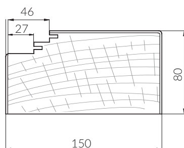
ROZŠÍRENIE PROFILU OBLOŽKOVEJ ZÁRUBNE K DVERÁM AKUSTIK A4 42dB OD 150 DO 370 mm
