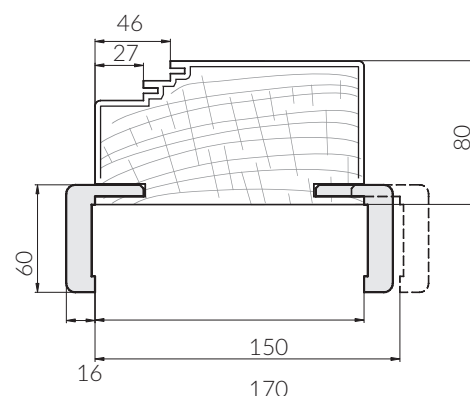
ROZŠÍRENIE PROFILU OBLOŽKOVEJ ZÁRUBNE K DVERÁM AKUSTIK A4 42dB OD 150 DO 370 mm
