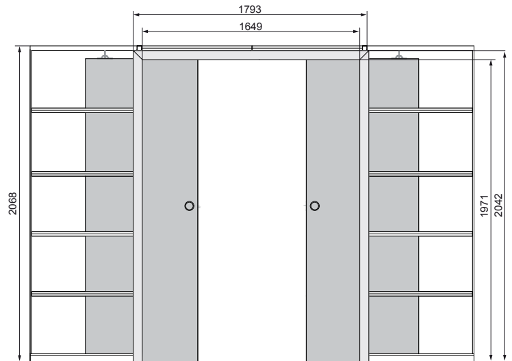
ZÁRUBEŇ ROZSAH 125 - STÁLÝ / ZÁRUBŇA ROZSAH 125 - STÁLÝ
