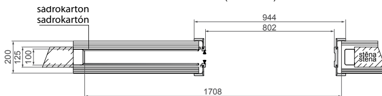
Zárubeň rozsah / Zárubňa rozsah (126-200) – SYMETRICKÁ*
