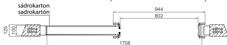
Zárubeň rozsah 125 - stály / Zárubňa rozsah 125 - stály
