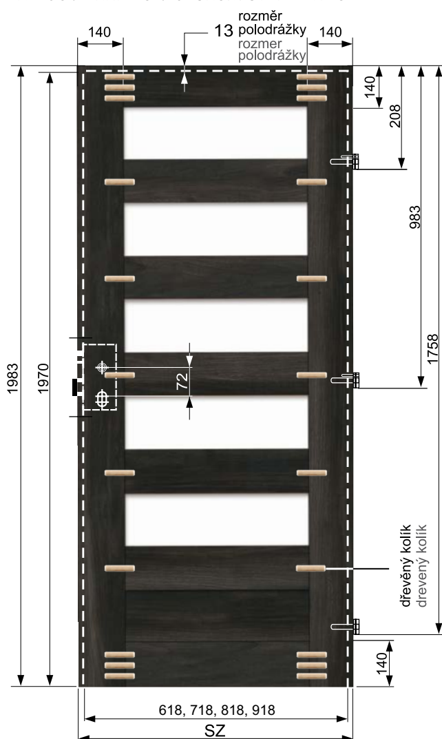
FALCOVÉ KŘÍDLO V ČESKÉM STANDARDU / FALCOVÉ KRÍDLO V ČESKOM ŠTANDARDU
