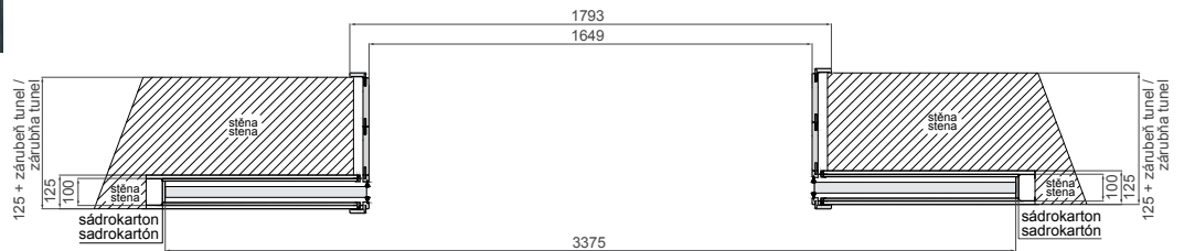
ZÁRUBEŇ ROZSAH / ZÁRUBŇA ROZSAH (200-220) DO (400-420) – ASYMETRICKÁ
