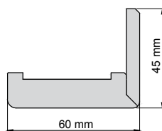
Úhelník pro nastavitelnou zárubeň - šířka 60 mm / Uholník pre nastaviteľnú zárubňu - šířka 60 mm
