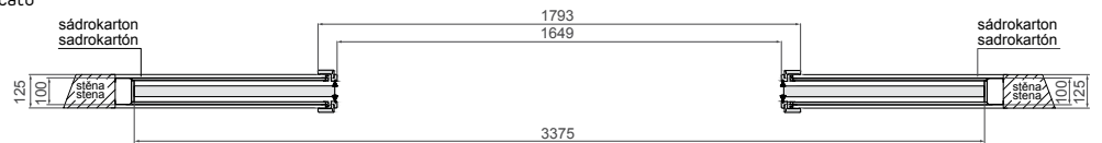
ZÁRUBEŇ ROZSAH / ZÁRUBŇA ROZSAH (126-200) – SYMETRICKÁ*
