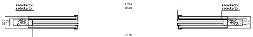
ZÁRUBEŇ ROZSAH / ZÁRUBŇA ROZSAH (126-200) – SYMETRICKÁ*
