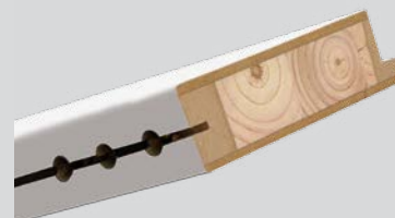
Litá - masivní RÁMOVÁ konstrukce / Lita - masívna RÁMOVÁ konštrukcia
