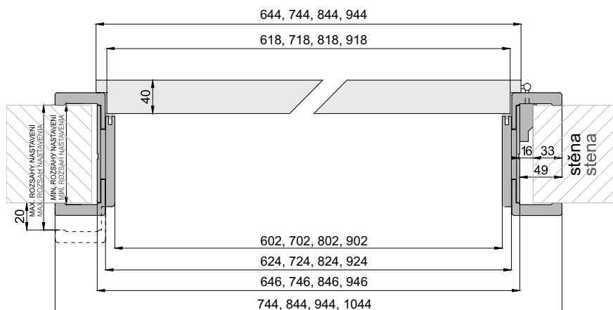
Úhelník pro nastavitelnou zárubeň - šířka 80 mm / Uholník pre nastaviteľnú zárubňu - šířka 80 mm
