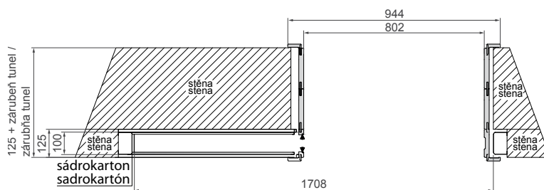
Zárubeň rozsah / Zárubňa rozsah (200-220) DO (400-420) – ASYMETRICKÁ
