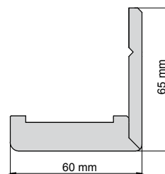
Úhelník rozšiřující pro nastavitelnou zárubeň - šířka 60 mm / Uholník rozšiřující pre nastaviteľnú zárubňu - šířka 60 mm
