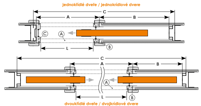
dvoukřídlé dveře / dvojkřídlové dveře
